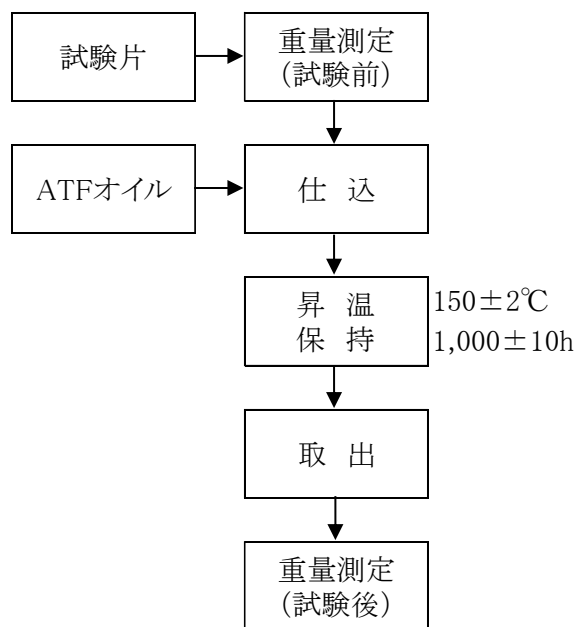
試験フロー
