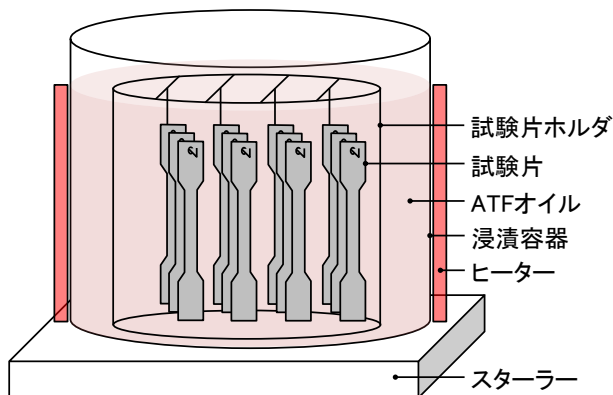
試験装置の構成
