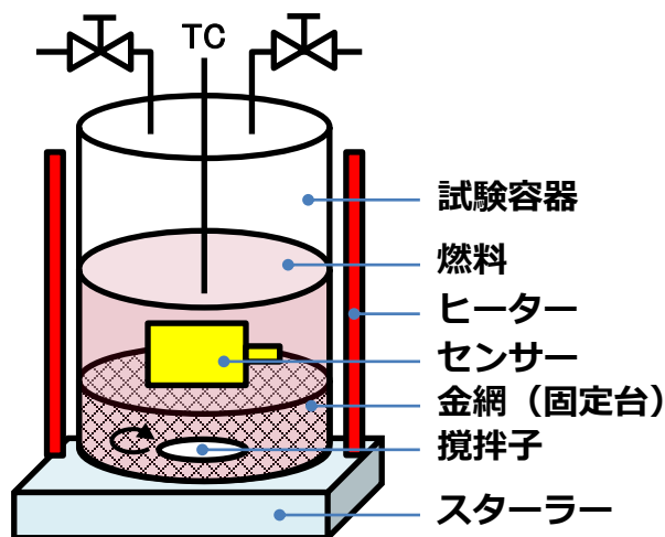
試験装置図
