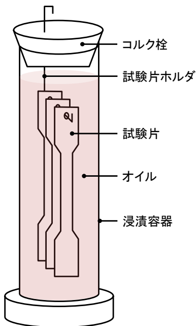
試験装置の構成
