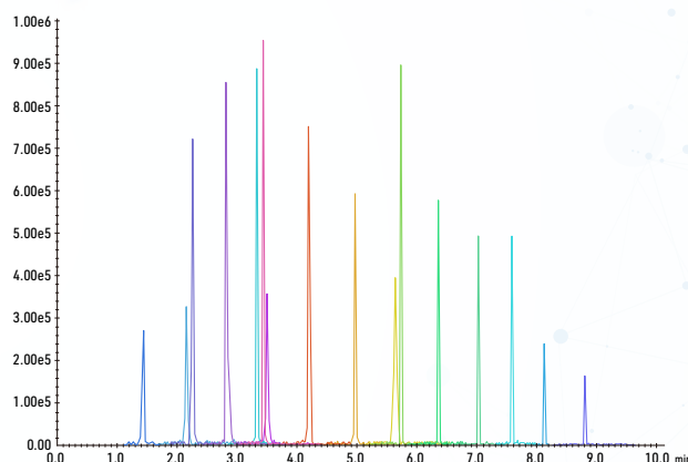
PFASのクロマトグラム例
