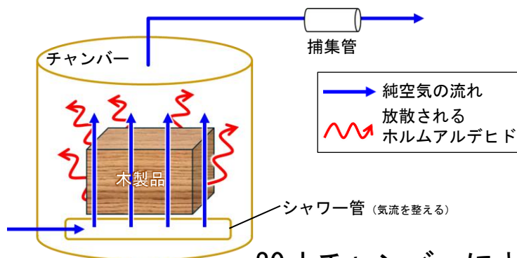
20 Lチャンバーによるホルムアルデヒド放散試験のイメージ
